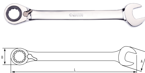
KLUCZ PŁASKO-OCZKOWY Z GRZECHOTKĄ I PRZEŁĄCZNIKIEM ZMIANY KIERUNKU
