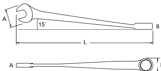
KLUCZ PŁASKO-OCZKOWY XL X-BEAM METRYCZNY
